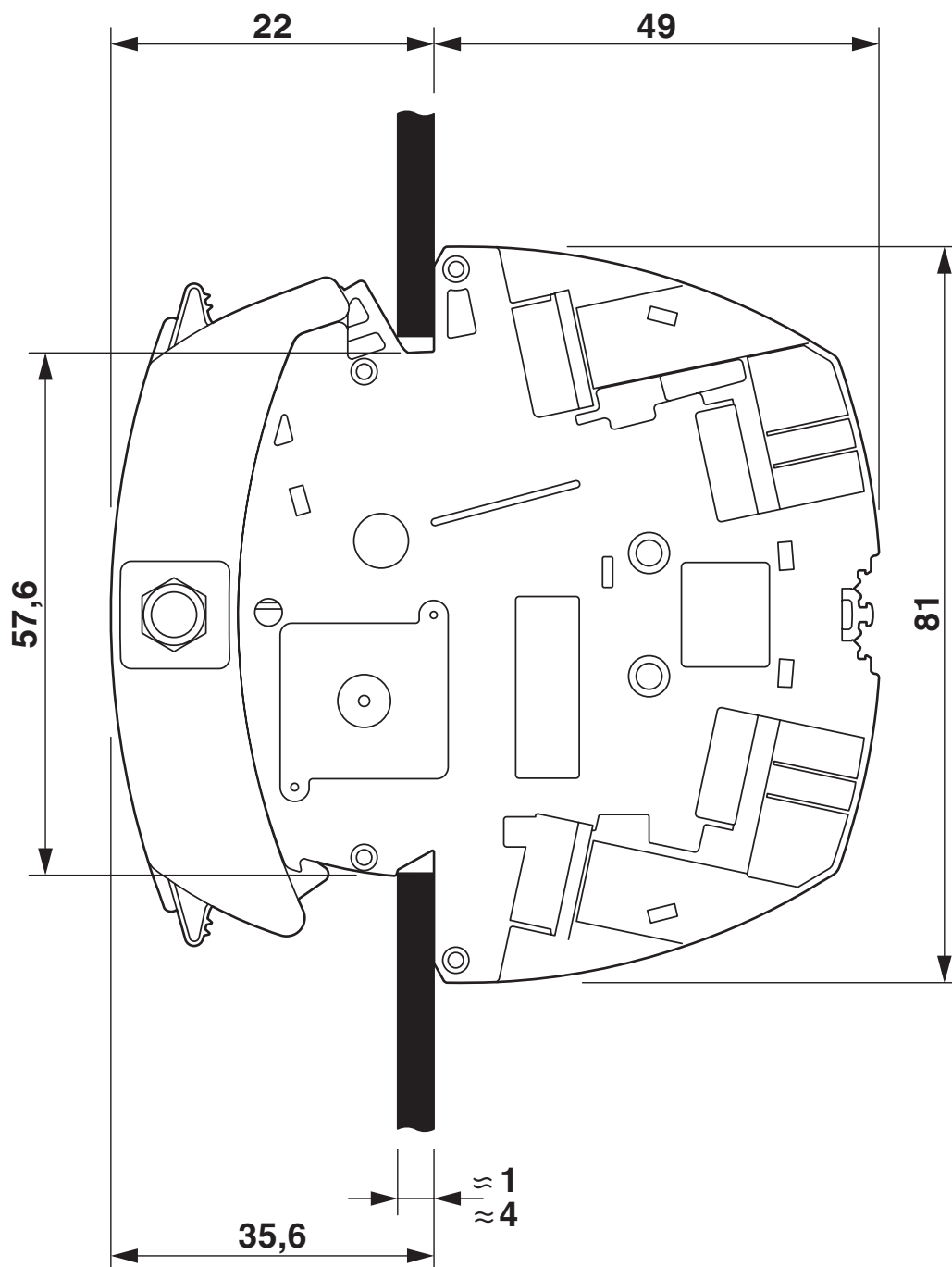
Rysunek wymiarowy
