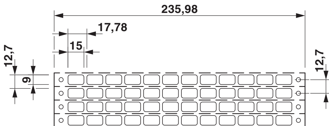
Rysunek wymiarowy
