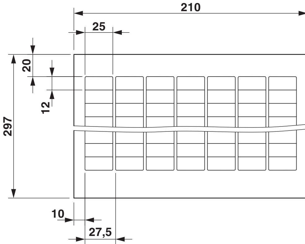
Rysunek wymiarowy
