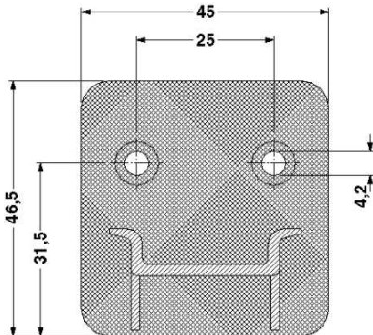
Rysunek wymiarowy
