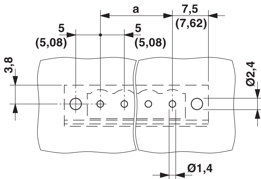
Rysunek wymiarowy
