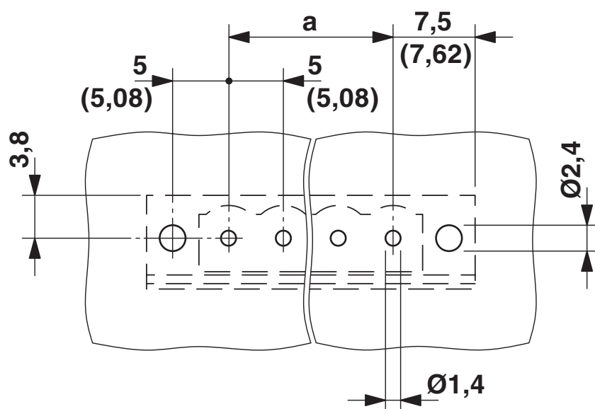
Rysunek wymiarowy
