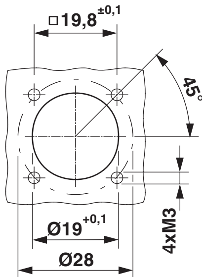
Rysunek wymiarowy
