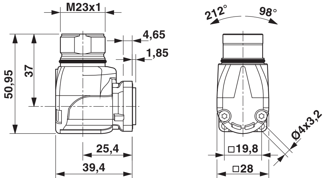
Rysunek wymiarowy
