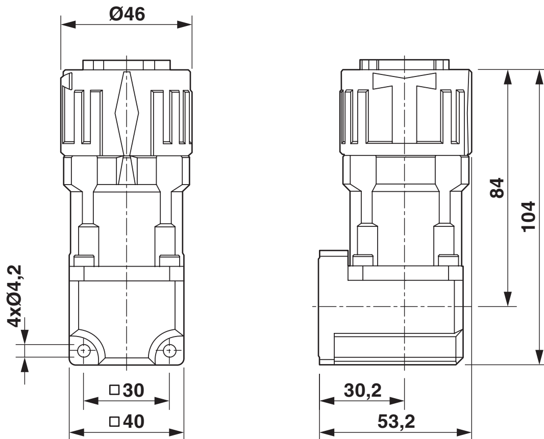
Rysunek wymiarowy
