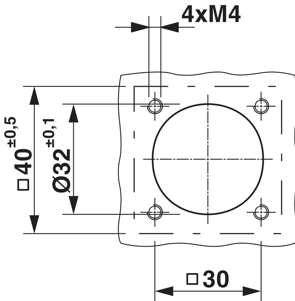
Rysunek wymiarowy
