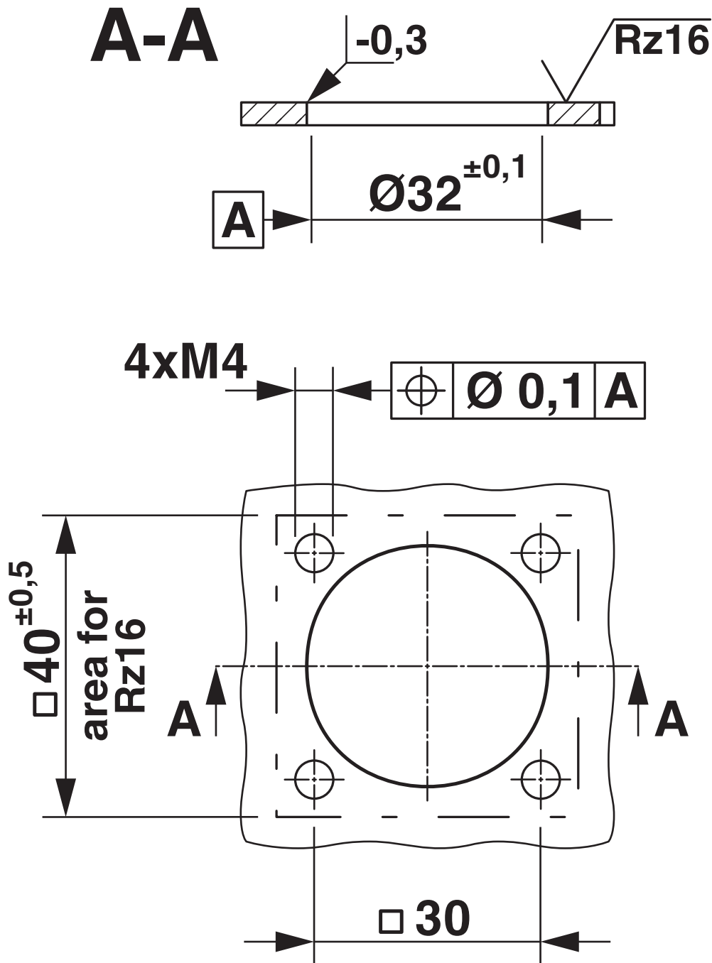
Rysunek wymiarowy
