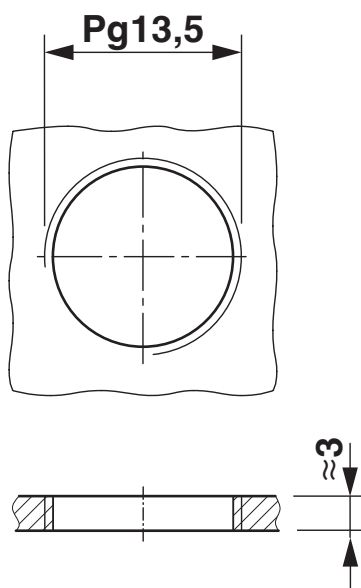
Rysunek wymiarowy
