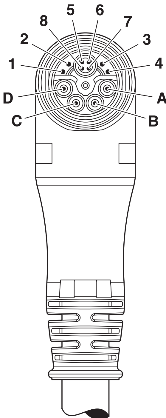
Rysunek schematyczny
