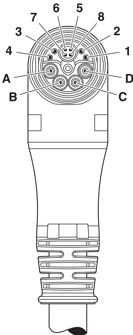
Rysunek schematyczny
