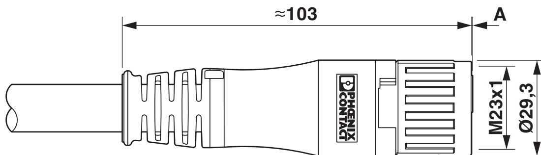
Rysunek wymiarowy
