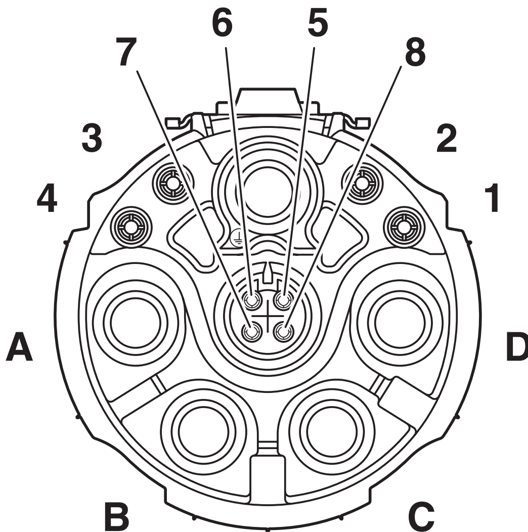
Układ styków złącza żeńskiego sygnałowego, kodowanie 2
