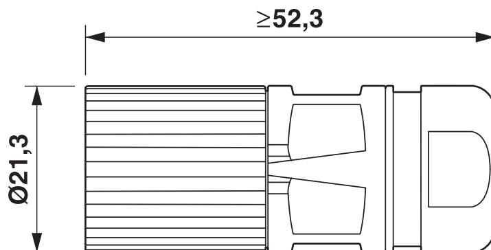
Rysunek wymiarowy
