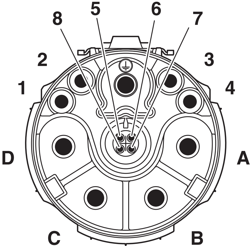
Rysunek schematyczny
