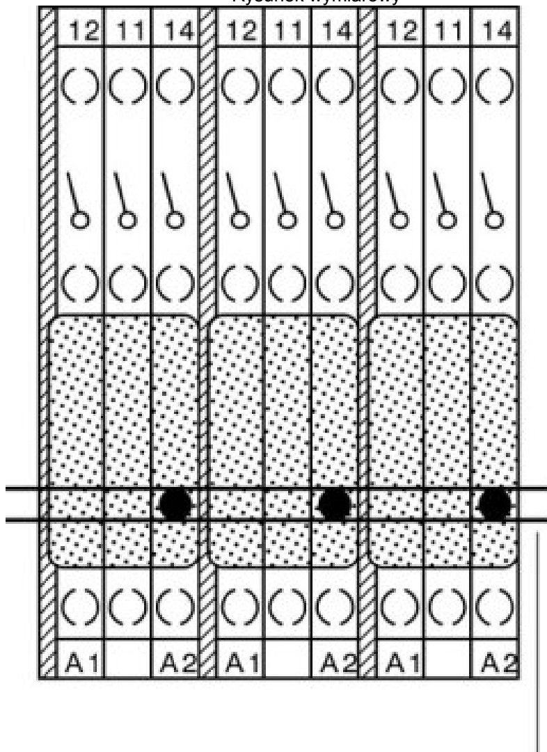
Rysunek wymiarowy
