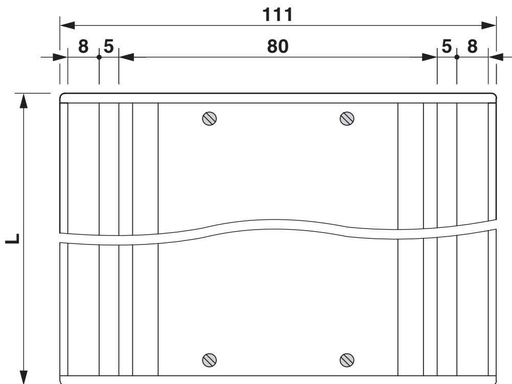
Rysunek wymiarowy
