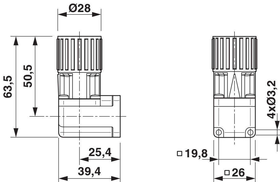
Rysunek wymiarowy
