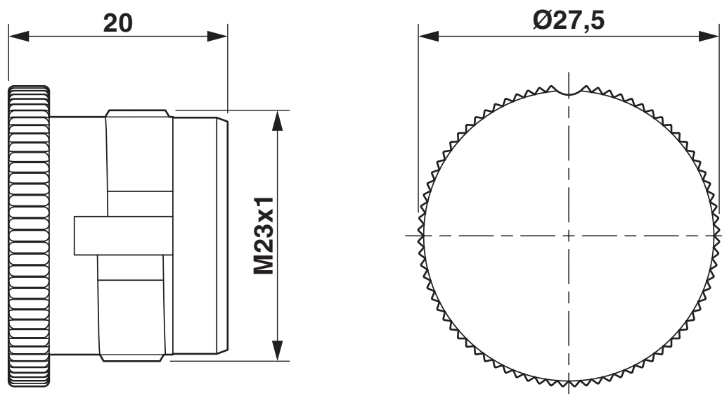
Rysunek wymiarowy
