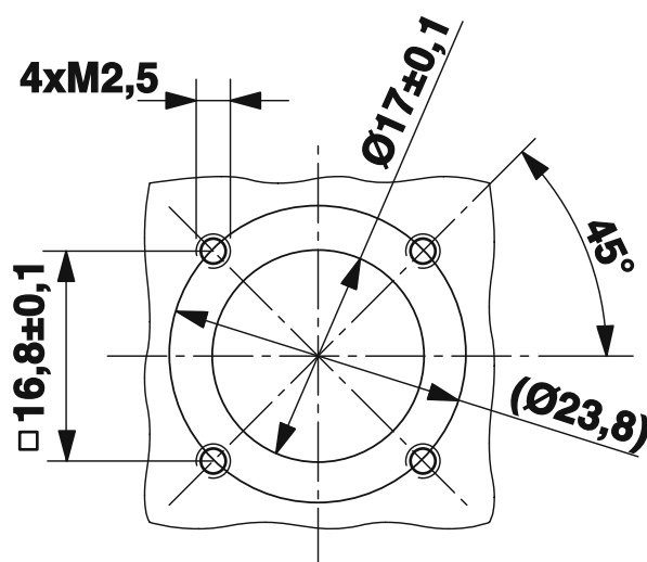
Rysunek wymiarowy
