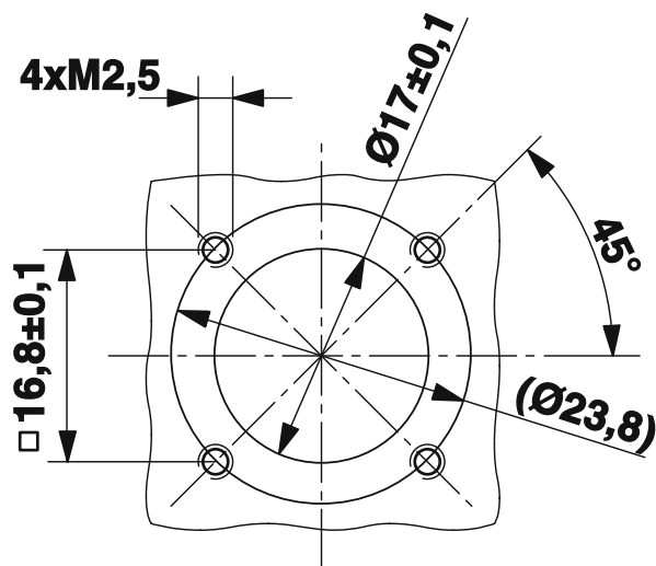
Rysunek wymiarowy
