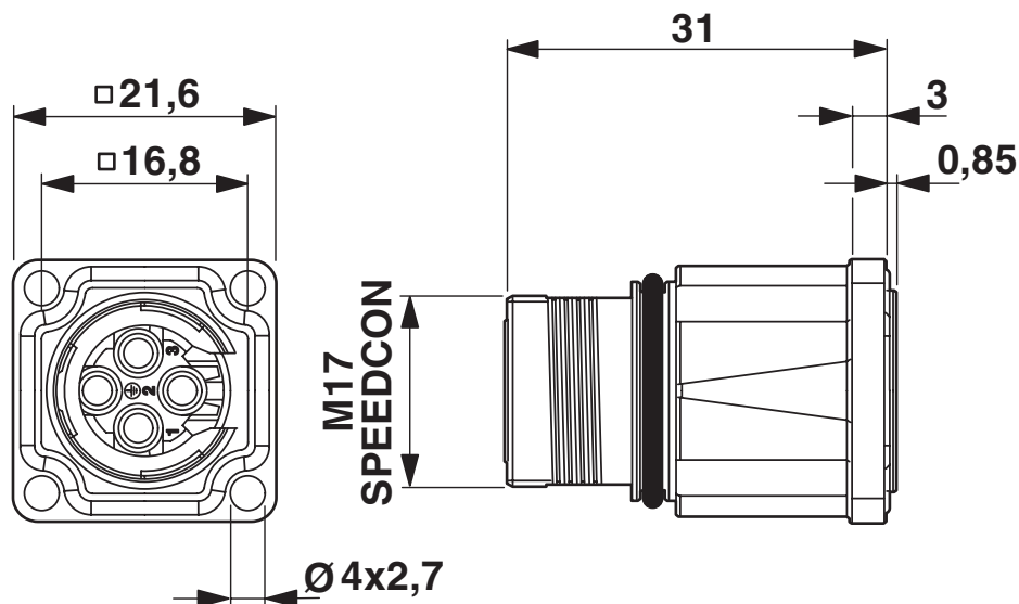
Rysunek wymiarowy
