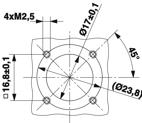
Rysunek wymiarowy
