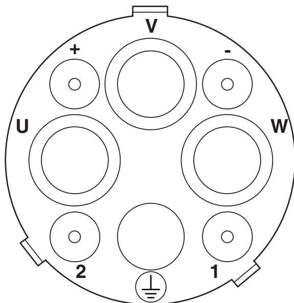
Rysunek schematyczny
