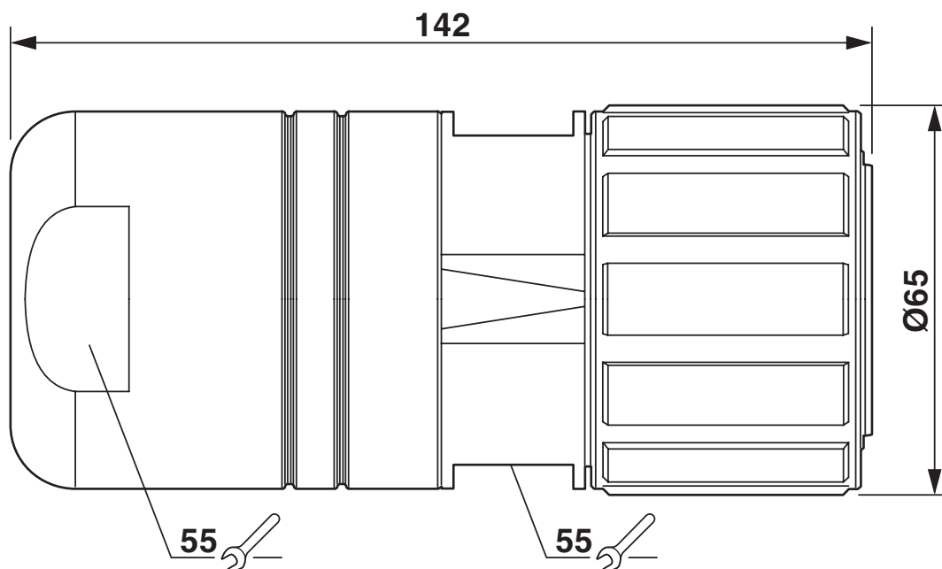
Rysunek wymiarowy
