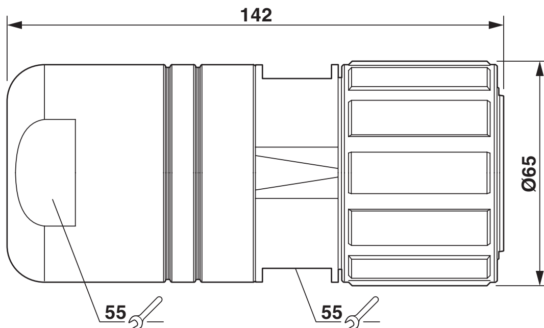
Rysunek wymiarowy
