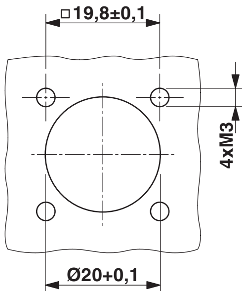
Rysunek wymiarowy
