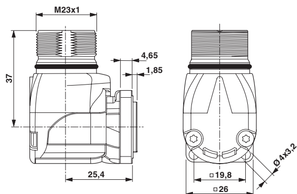
Rysunek wymiarowy
