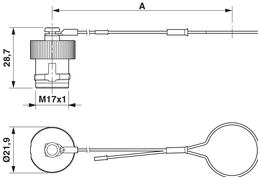
Rysunek wymiarowy
