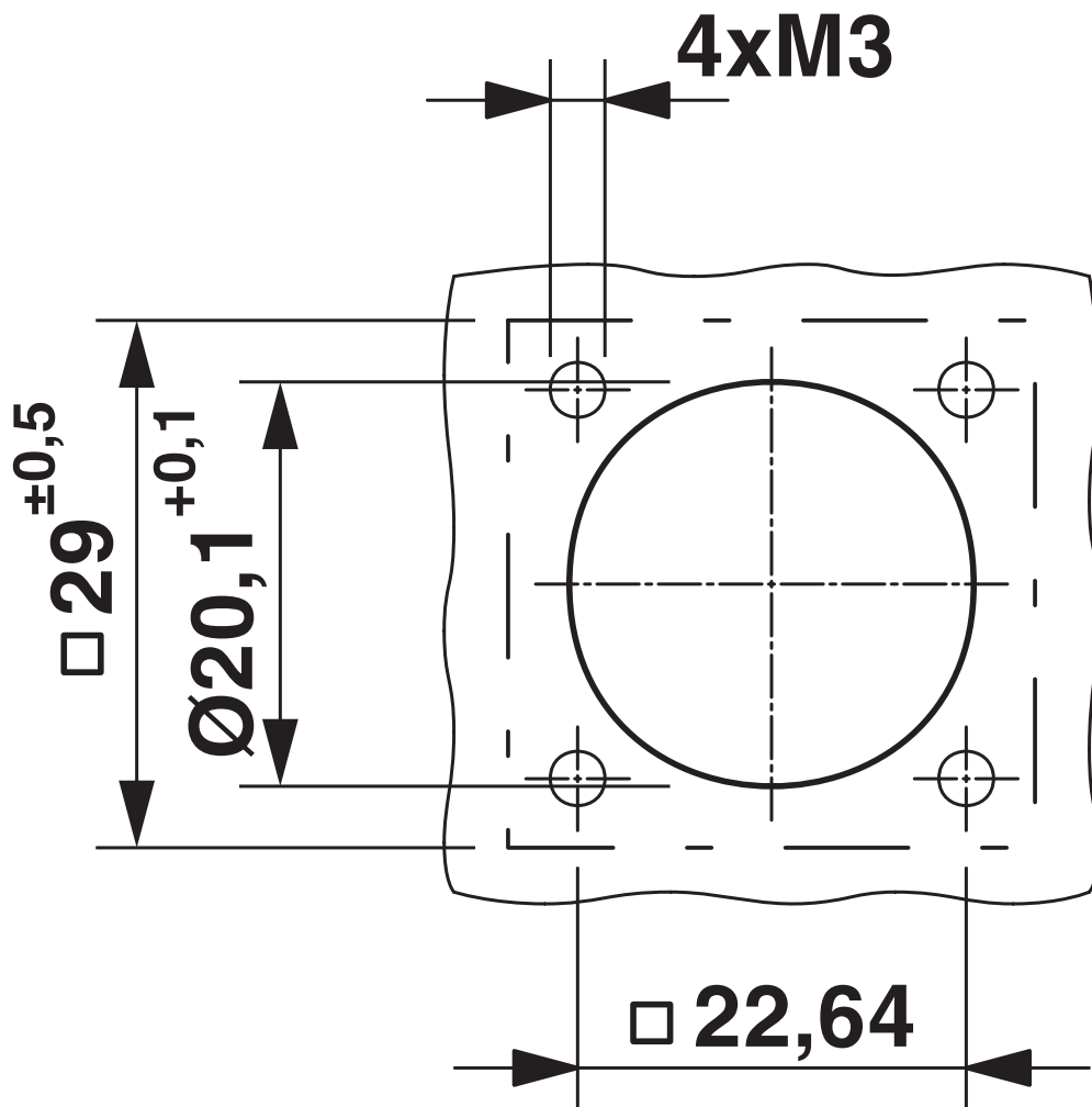
Rysunek wymiarowy
