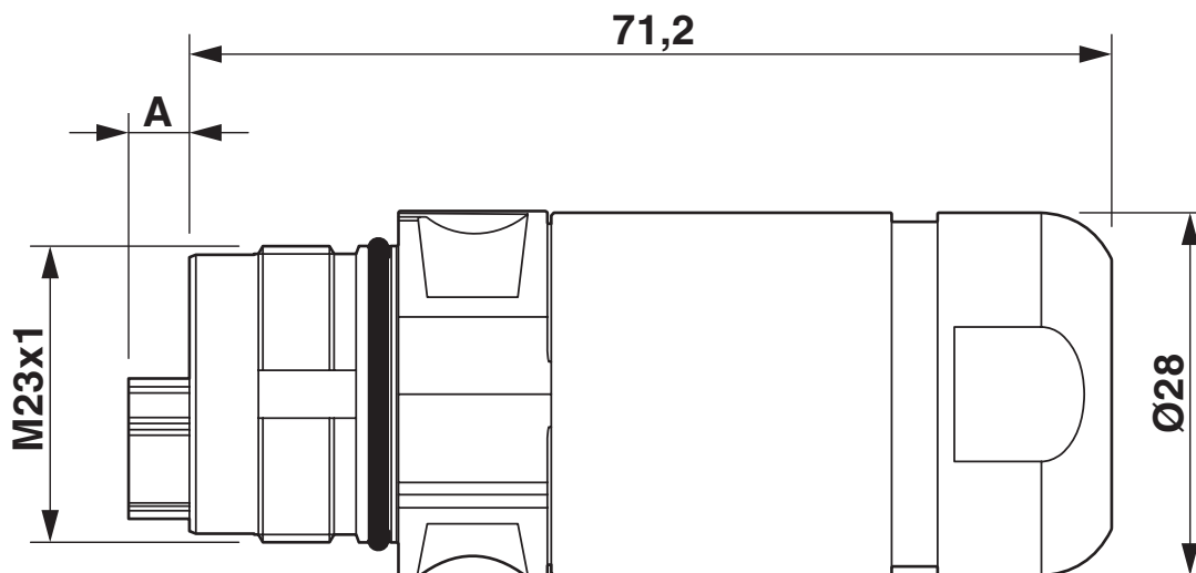
Rysunek wymiarowy
