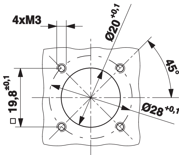
Rysunek schematyczny
