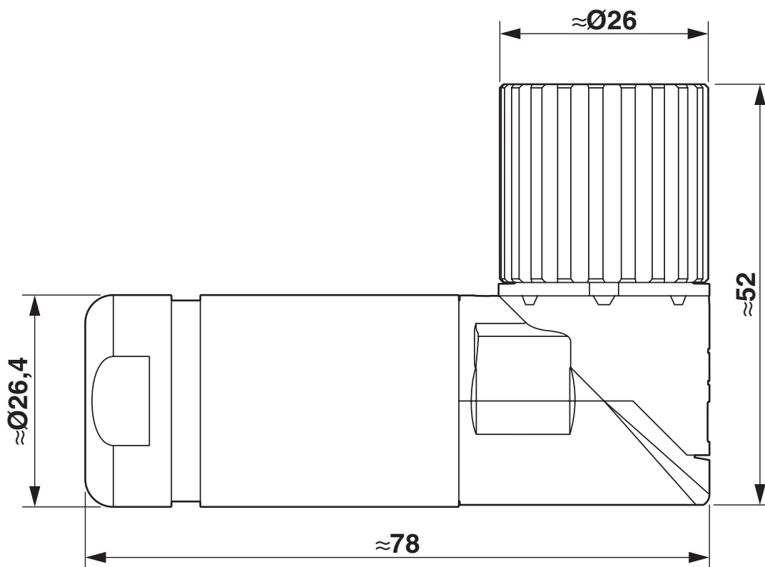
Rysunek wymiarowy
