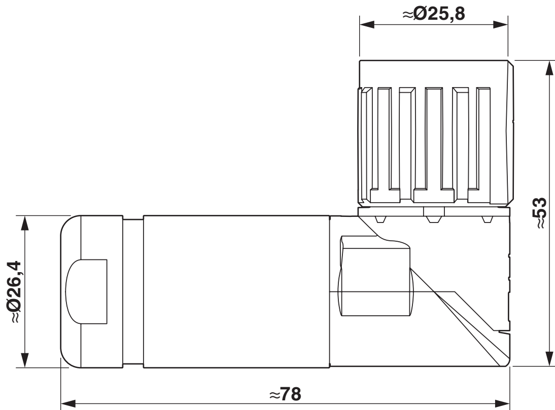
Rysunek wymiarowy
