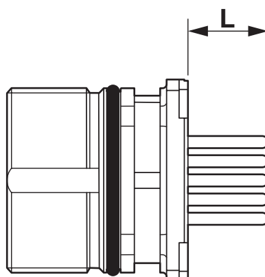
Rysunek wymiarowy
