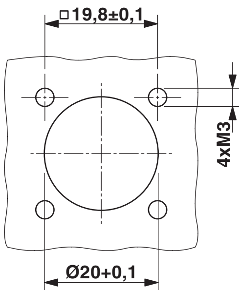
Rysunek wymiarowy
