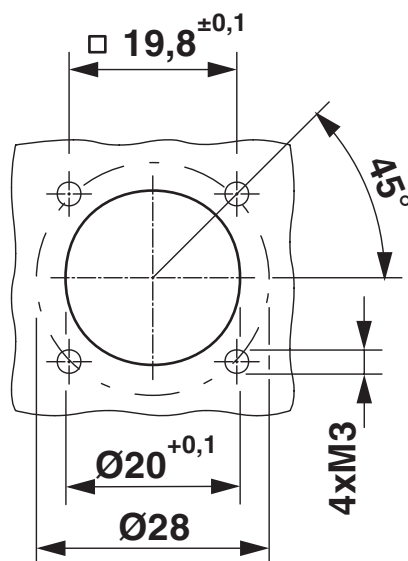
Rysunek schematyczny
