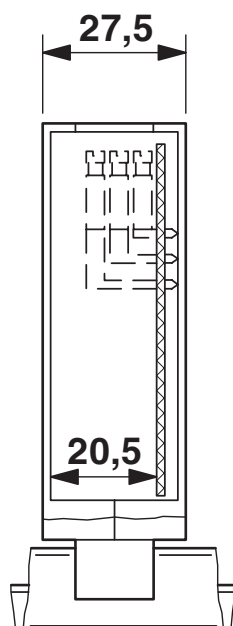
Rysunek wymiarowy
