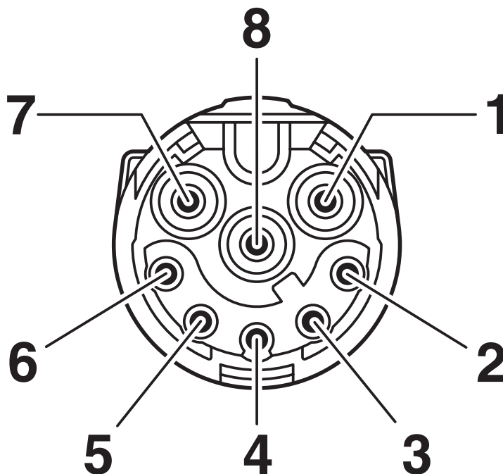
Rysunek schematyczny
