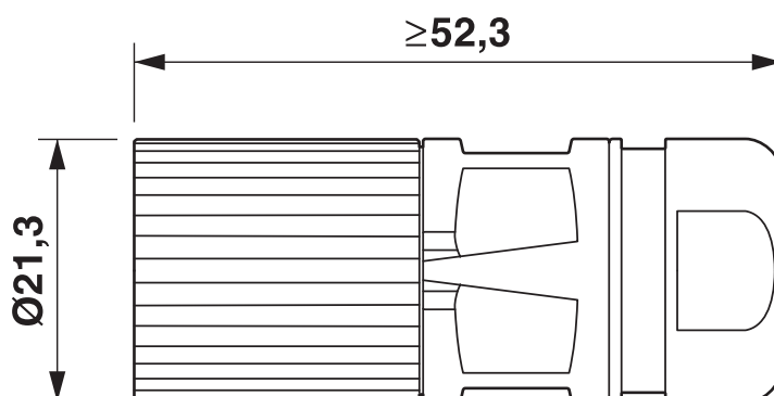
Rysunek wymiarowy
