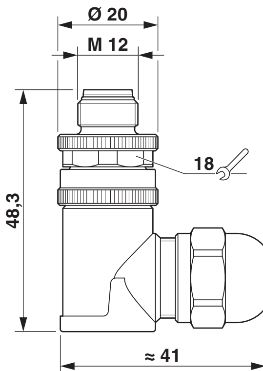
Rysunek wymiarowy
