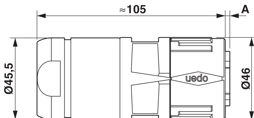
Rysunek wymiarowy
