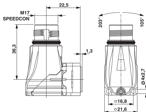
Rysunek wymiarowy
