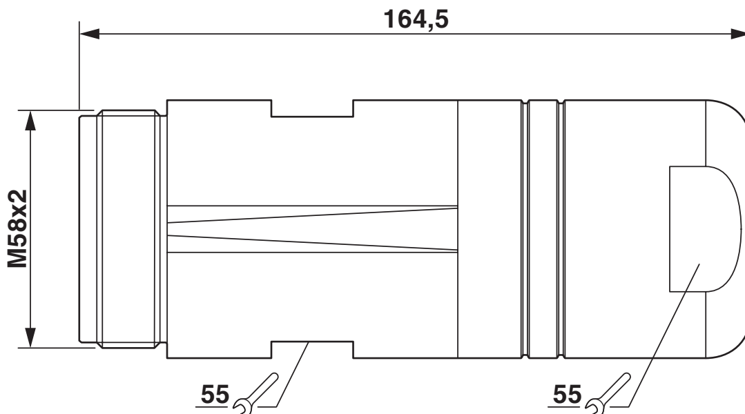
Rysunek wymiarowy
