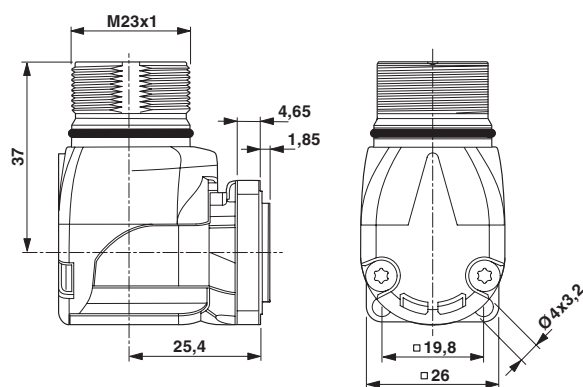
Rysunek wymiarowy
