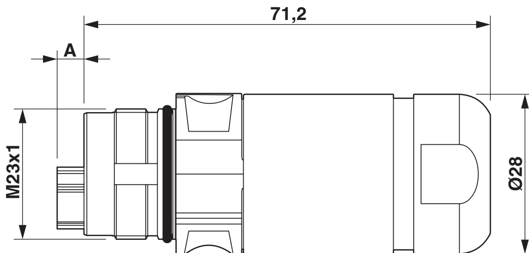
Rysunek wymiarowy
