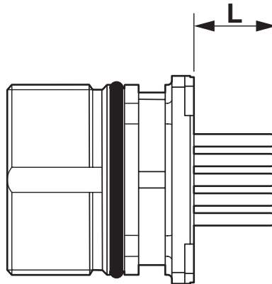
Rysunek wymiarowy
