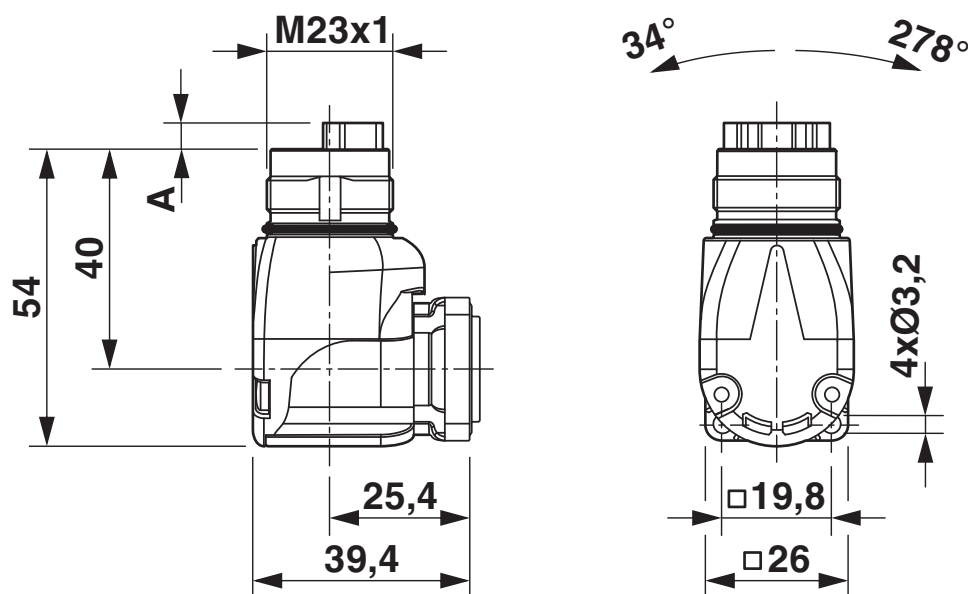
Rysunek wymiarowy
