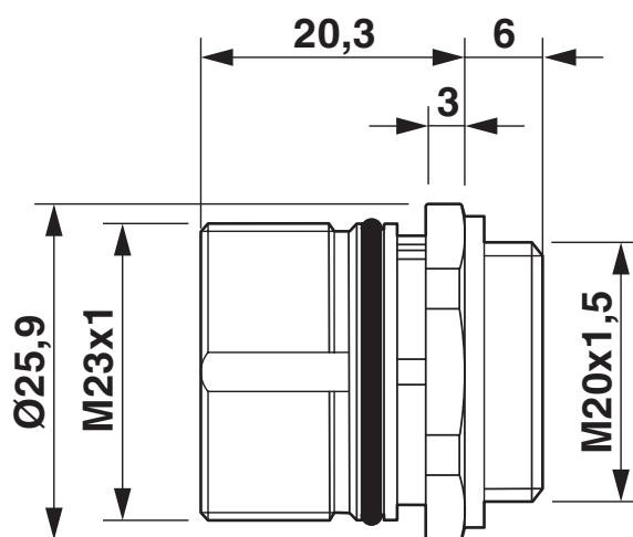
Rysunek wymiarowy
