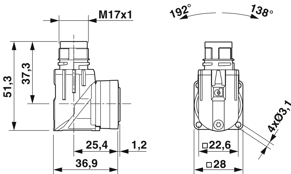
Rysunek wymiarowy
