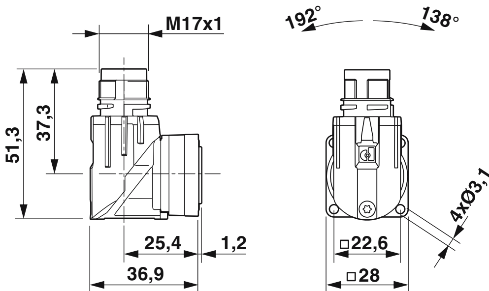
Rysunek wymiarowy
